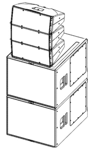
d&b T-Series T10/ B4-SUB グランドスタック
